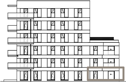
GEVEL OOST
