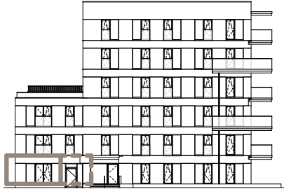
GEVEL WEST
