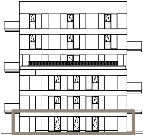
GEVEL NOORD
